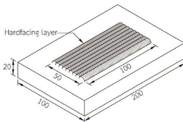
ก) ขอบเขตการเชื่อมพอกผิวแข็ง
