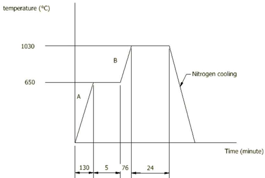
รูปที่ 2 อุณหภูมิและเวลาที่ใช้ในการทำการชุบผิวแข็งของเหล็กกล้าไร้สนิม AISI 420 ที่ 1,030°C
