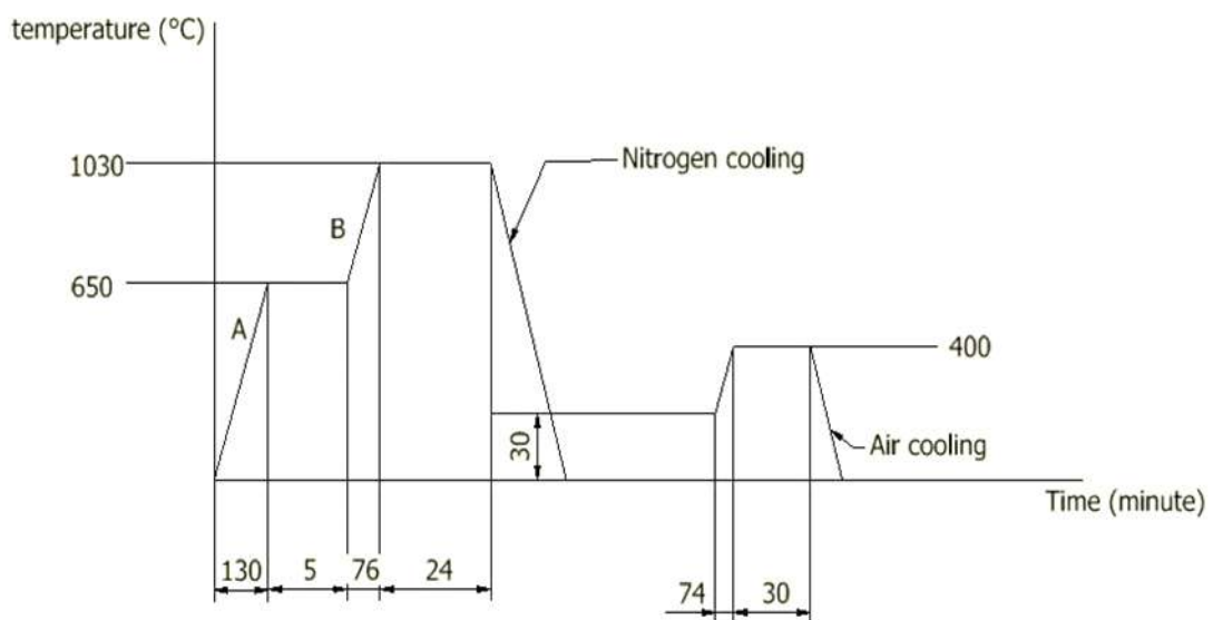
รูปที่ 3 อุณหภูมิและเวลาที่ใช้ในการทำการอบคืนตัวของเหล็กกล้าไร้สนิม AISI 420 ที่ 1,030°C
