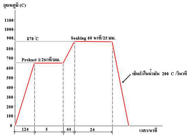
ข. กราฟอุณหภูมิการชุบผิวแข็ง
