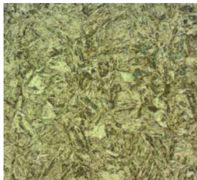
รูปที่ 12 โครงสร้างของเหล็กกล้าไร้สนิม AISI 420 ที่ผ่านการอบคืนตัว โดยใช้เวลาในการอัด 9 s และความดันในการอัด 30 MPa
