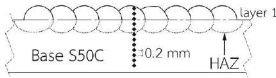
รูปที่ 3 ทิศทางการทดสอบความแข็ง
