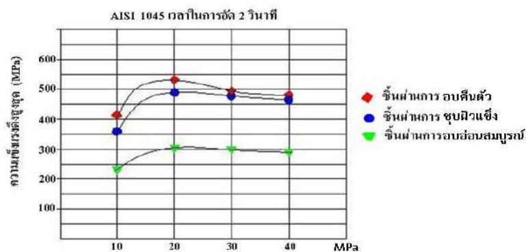
รูปที่ 6 ผลการเปรียบเทียบแรงดึงสูงสุดขึ้นงานตามเวลาในการอัด
