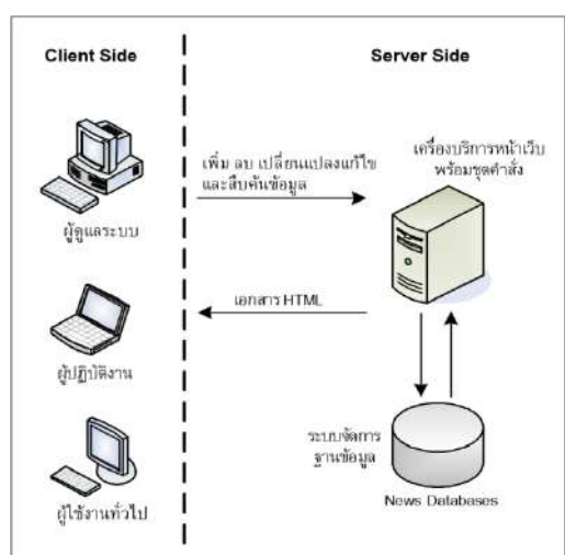
รูปที่ 1 สถาปัตยกรรมแบบทรีเทียร์
