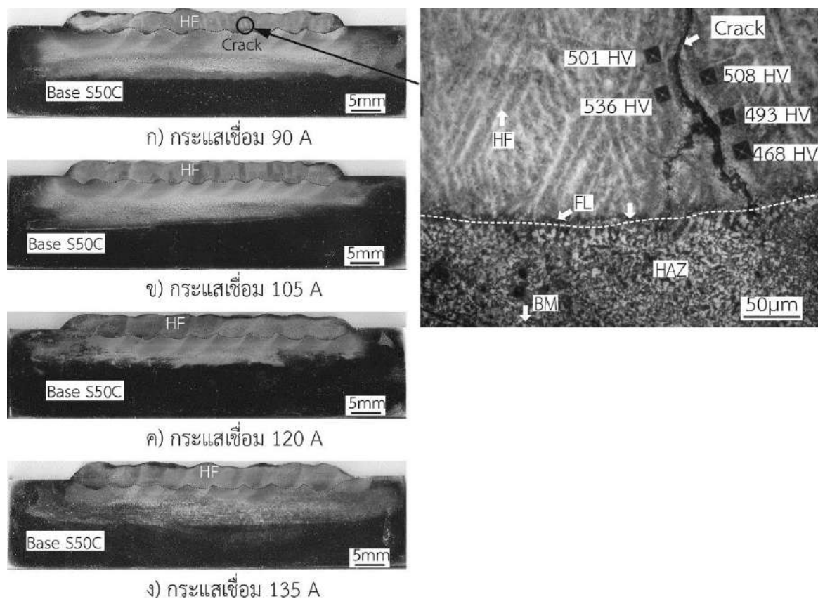
รูปที่ 5 โครงสร้างมหภาคโลหะเชื่อมพอกผิวแข็ง
