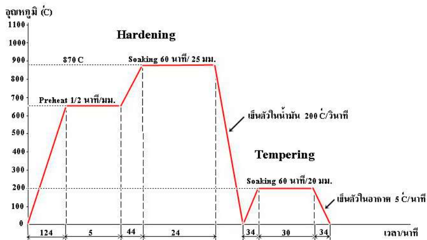
ค. กราฟอุณหภูมิการอบคืนตัว
