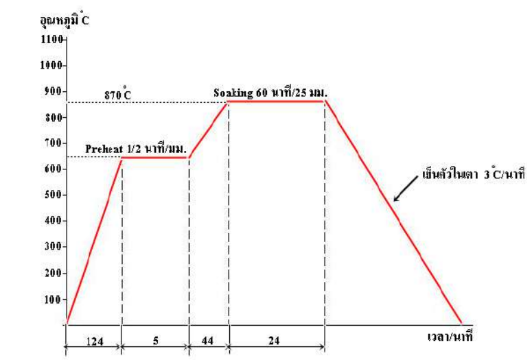
ก. กราฟอุณหภูมิการอบอ่อนสมบูรณ์
