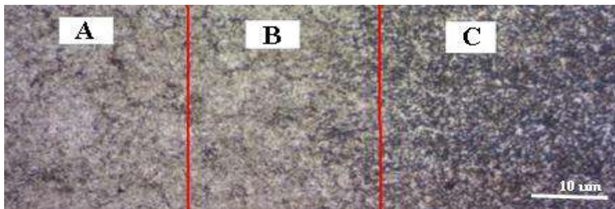
รูปที่ 11 โครงสร้างของเหล็กกล้าคาร์บอนปานกลาง AISI 1045 ที่ผ่านการอบอ่อนสมบูรณ์ ด้วยเวลาในการอัด 2 วินาทีและความดันในการอัด 2 MPa
