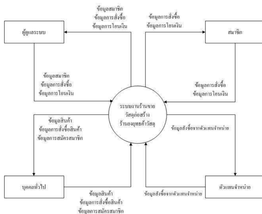
ภาพที่ 1 คอนเท็กซ์ไดอะแกรมระบบงานร้านยงยุทธคำวิสต์
