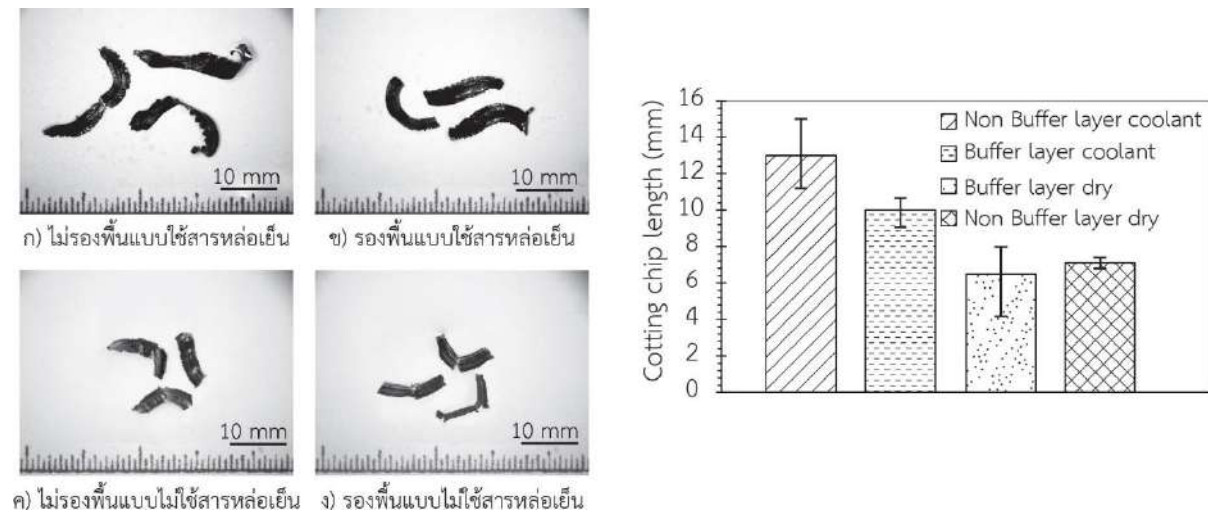
รูปที่ 5 รูปร่างลักษณะของเศษตัด
