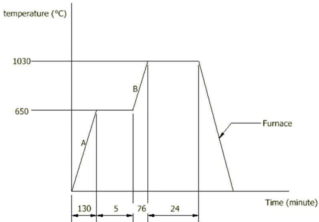
รูปที่ 1 อุณหภูมิและเวลาที่ใช้ในการทำการอบอ่อนสมบูรณ์ของเหล็กกล้าไร้สนิม AISI 420 ที่ 1,030^{\circ}\text{C}
