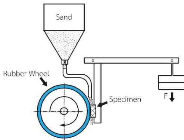
ก) เครื่องทดสอบ
