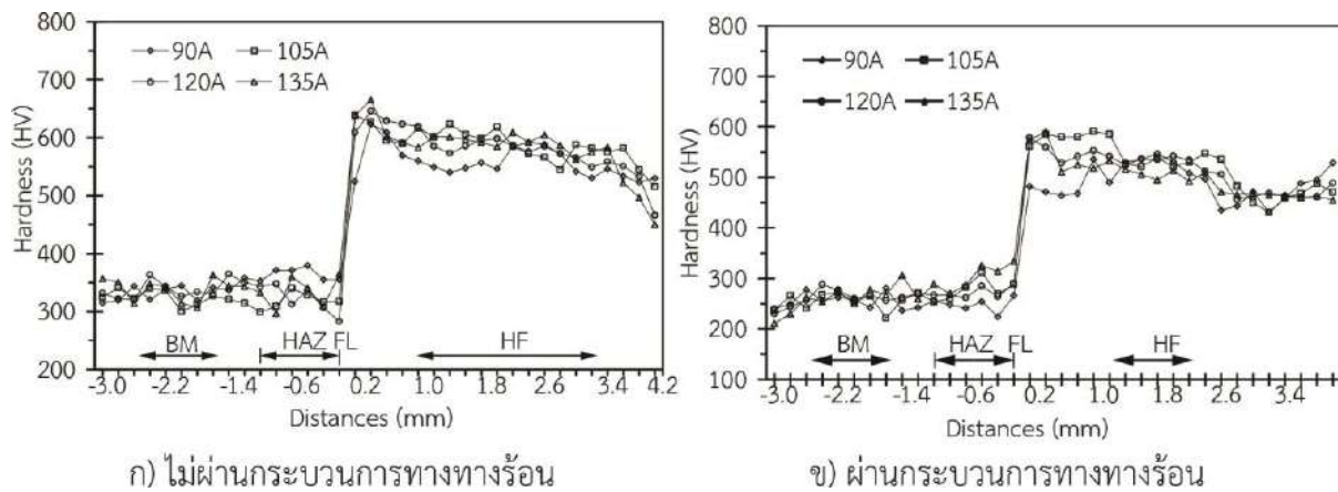
รูปที่ 6 การทดสอบค่าความแข็ง
