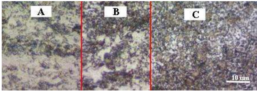
รูปที่ 11 โครงสร้างของเหล็กกล้าคาร์บอนปานกลาง AISI 1045 ที่ผ่านการอบอ่อนสมบูรณ์ ด้วยเวลาในการอัด 2 วินาทีและความดันในการอัด 2 MPa
