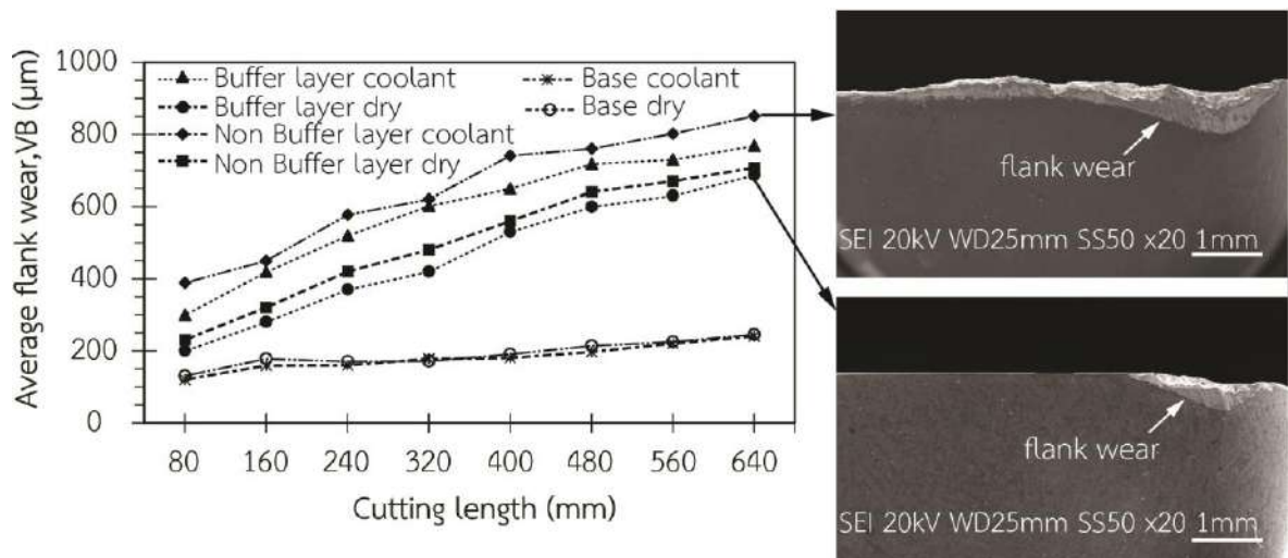
รูปที่ 6 ความสัมพันธ์ของระยะในการตัดเฉือนที่ส่งต่อการสึกหรอของคมตัด
