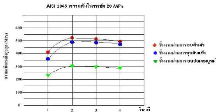
รูปที่ 5 ผลการเปรียบเทียบความแข็งแรงดึงสูงสุดขึ้นงานตามเวลาในการอัด
