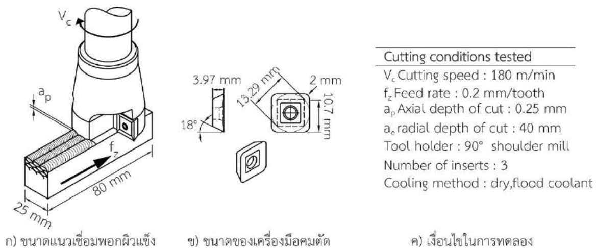
รูปที่ 2 กระบวนการกัดผิวหน้ารอยเชื่อม
