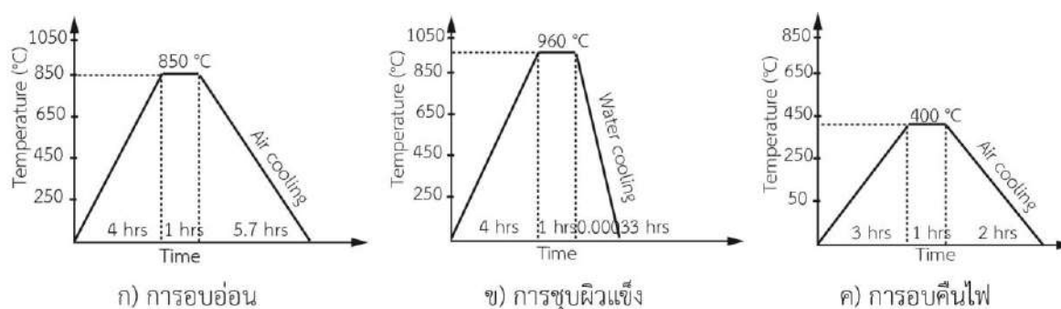
รูปที่ 2 กระบวนการทางความร้อน
