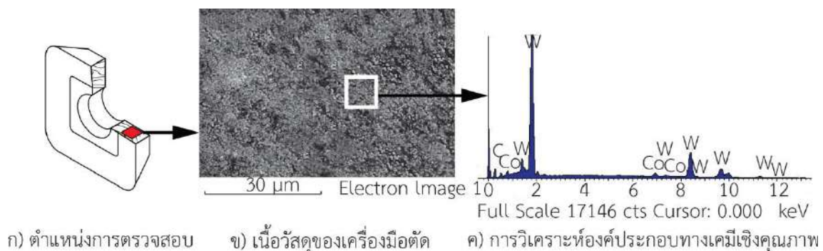
รูปที่ 3 การตรวจสอบส่วนผสมทางเคมีของเครื่องมือตัด
