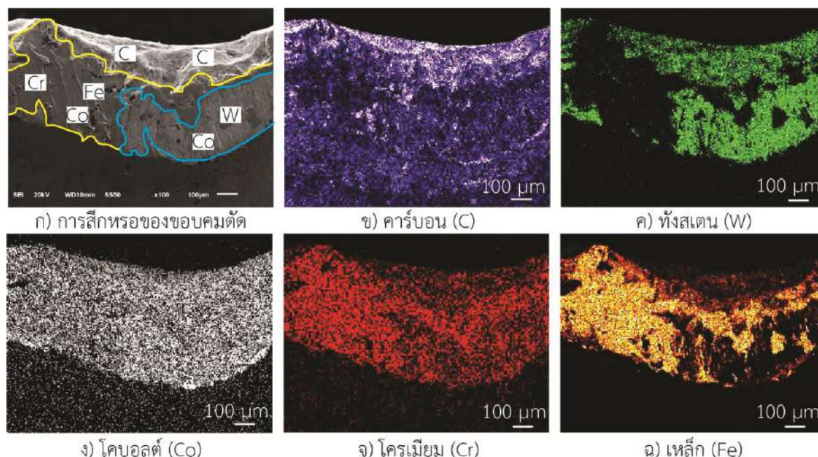
รูปที่ 8 แผนที่แถบรังสีการกระจายตัวพลังงาน (EDS maps) ขององค์ประกอบทางเคมีในการสึกหรอคมตัด
